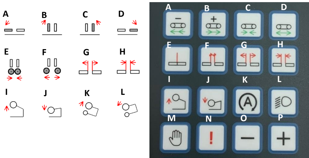
Tastenbelegung Notbedienung
