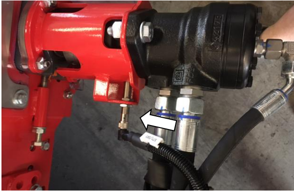
Induktiv-Sensor Banddrehzahl
